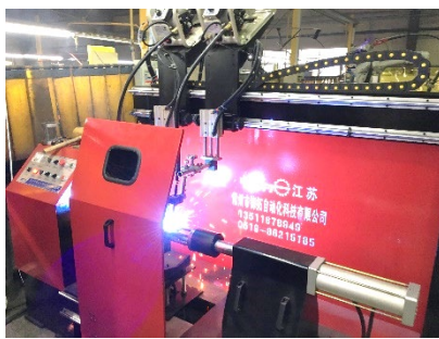
自動溶接機
